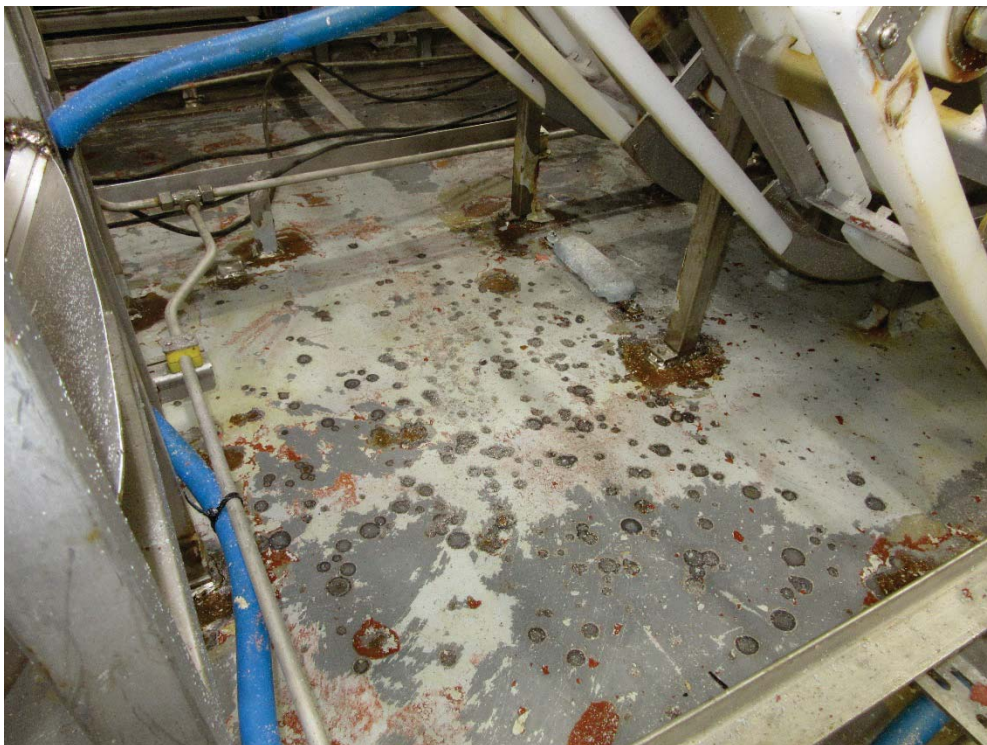
Figur 29. Umalt fabrikkdekk i karbonstål med korrosjonsangrep og anode med begrenset rekkevidde
